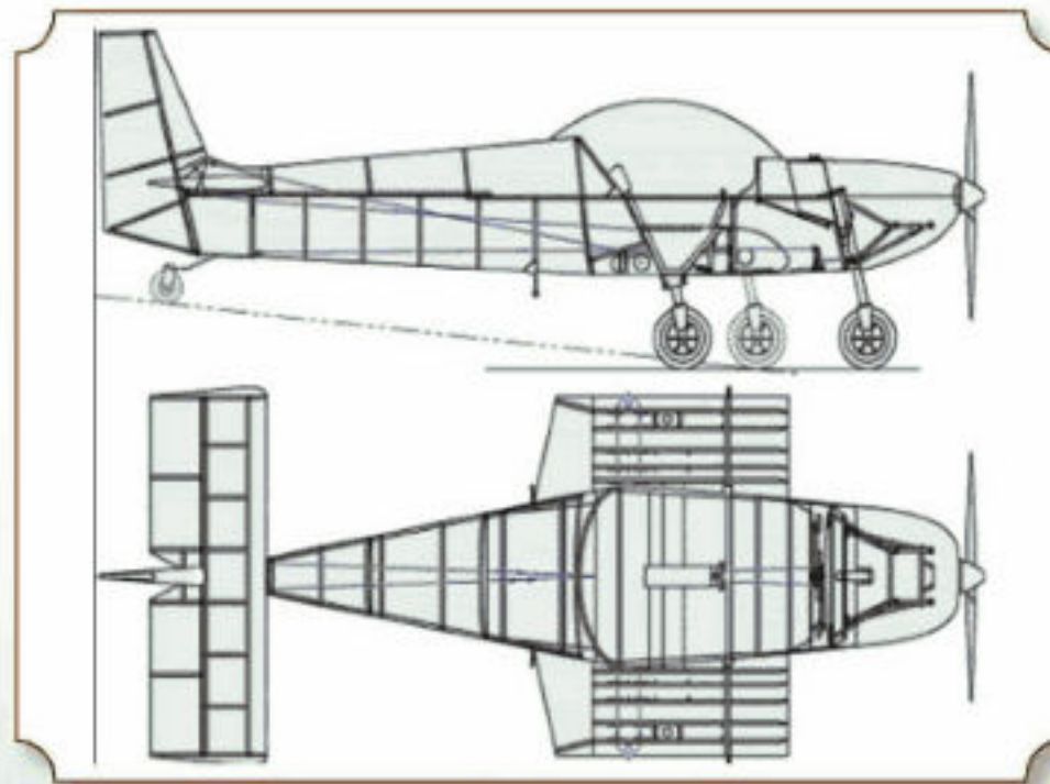
شكل (٦) تصميم.
